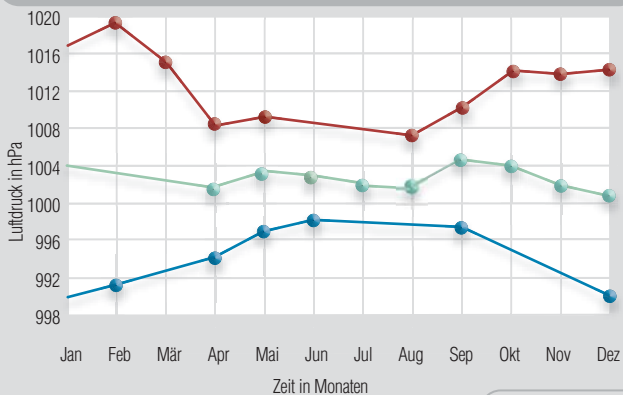
Luftdruck-Jahresdiagramm
