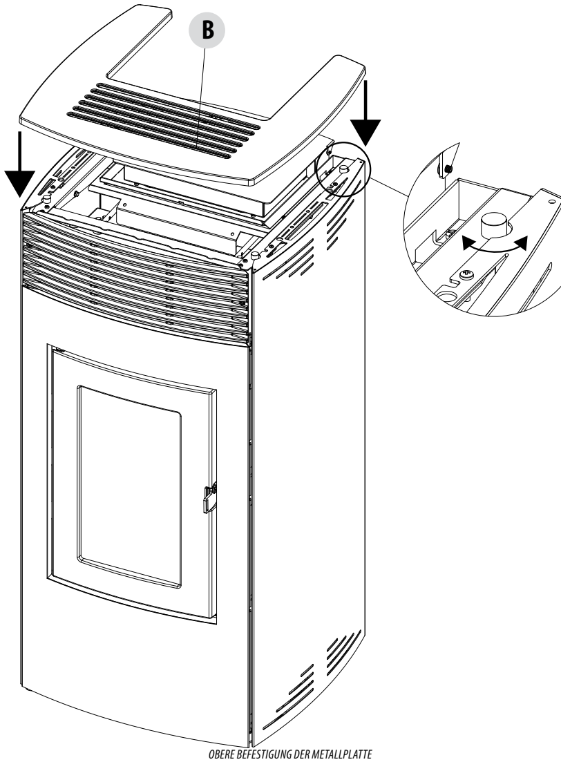
OBERE BEFESTIGUNG DER METALLPLATTE
