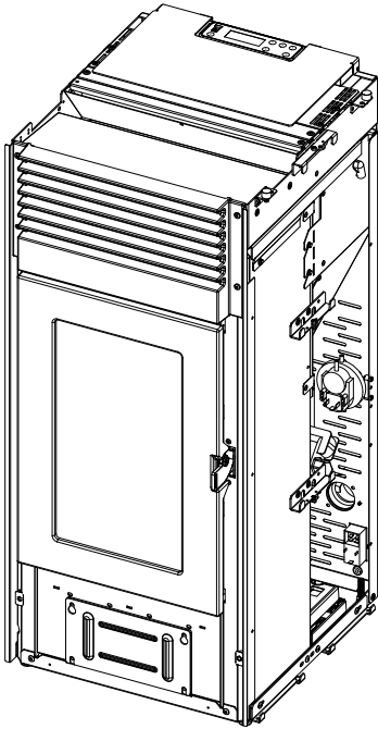
KAMINOFEN OHNE VERKLEIDUNG
