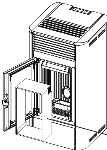
VERPACKUNG DES OFENS CAMEILA AUS STAHL
